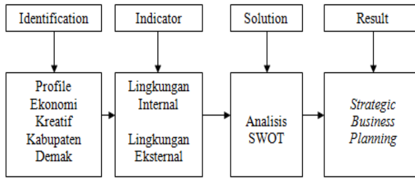
Gambar 1 Tahapan Penelitian
